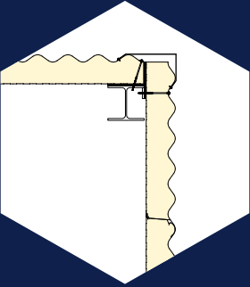
3. hoekdetail gevel
