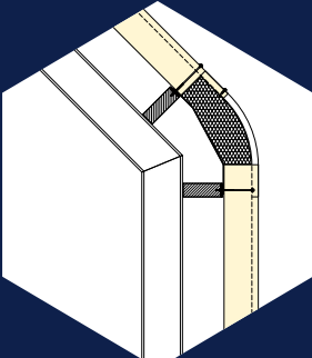
2. overgangsdetail dak/gevel
