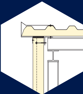
3. windveerdetail
